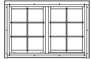
Nr. 14-2 Fönster 40 mm 1530 x 990 mm
