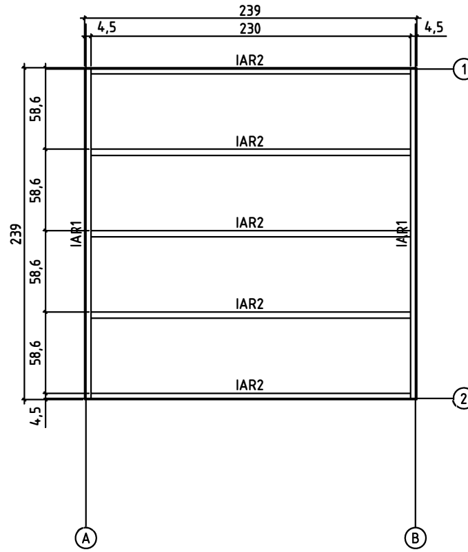
FOUNDATION - FUNDAMENT - FONDATION
